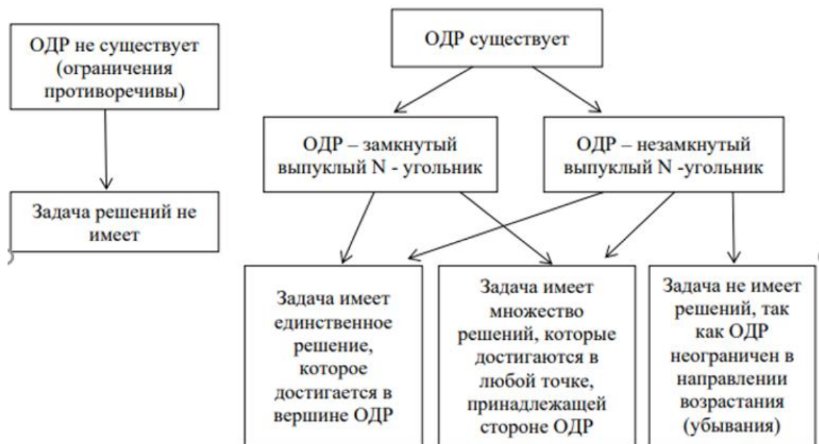
Рис. 5.1. Блок - схема
