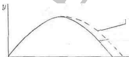
Рис. 5.0 - Траектория полета тела
