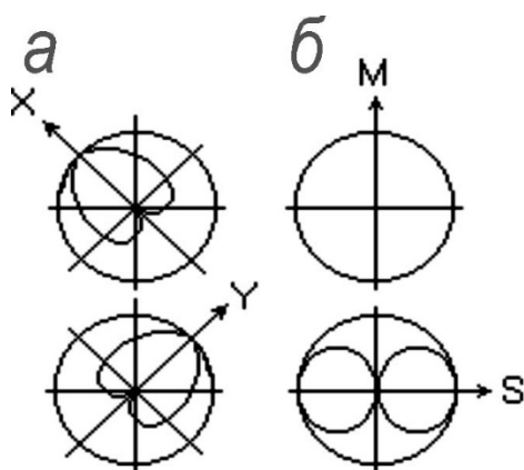
Рис.7.1. Характеристики направленности стереофонических микрофонов
