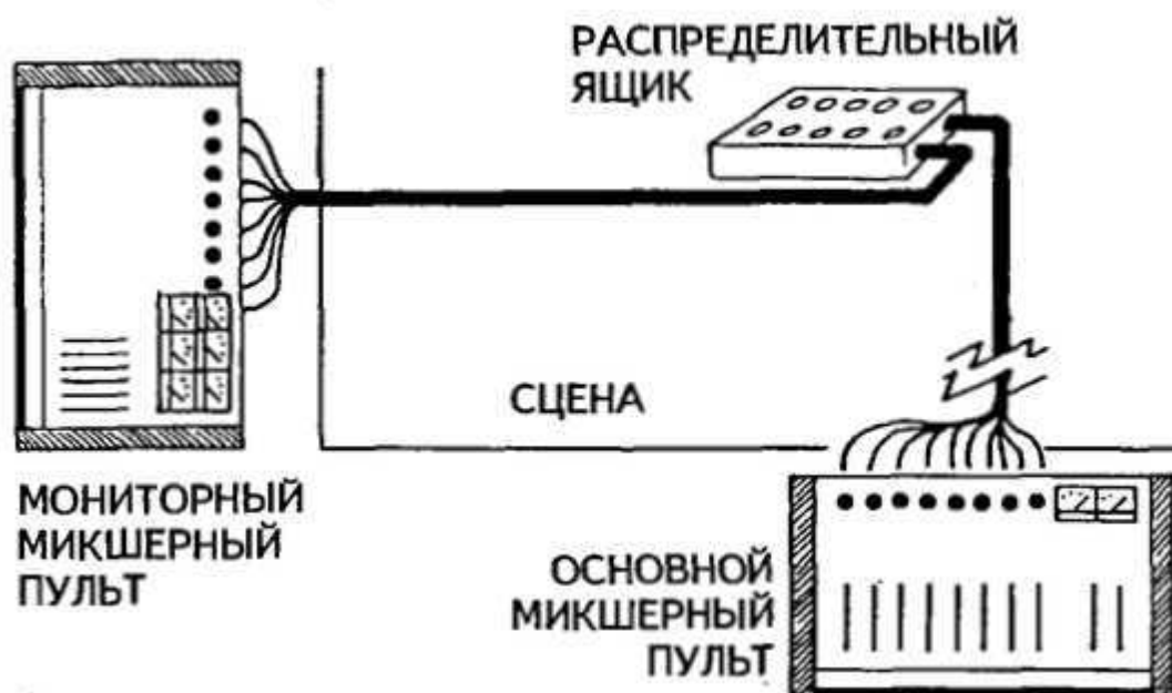
Рис. 6.1. Независимая мониторная система
